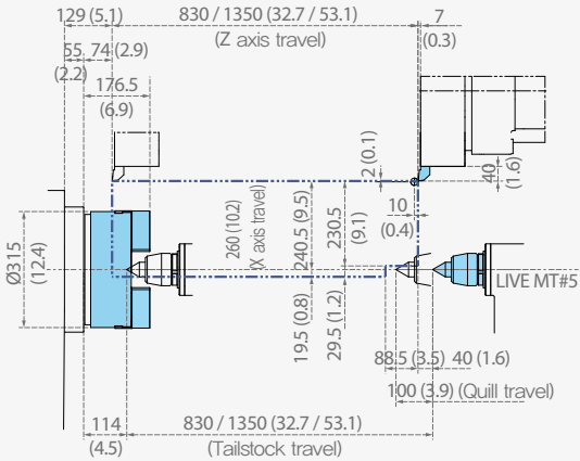
OD Holder
